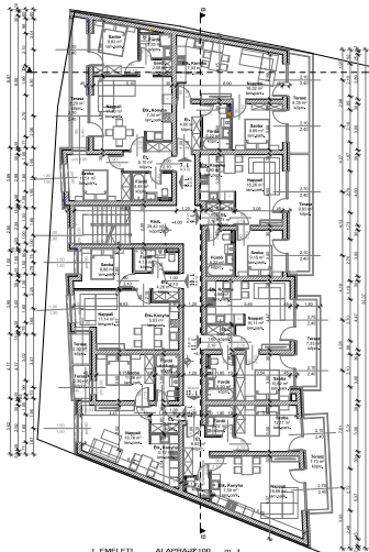
I. EMELETT ALAPRAJZ 100
