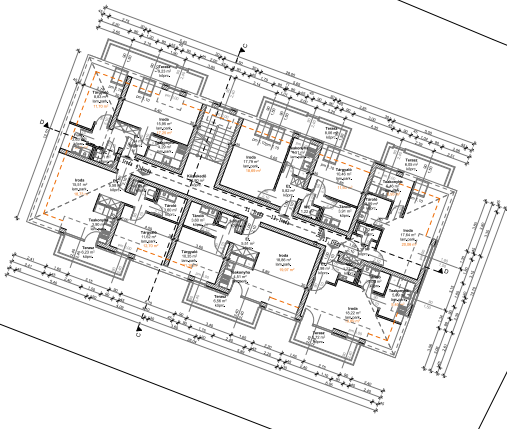
I. EMELETT ALAPRAJZ 100
