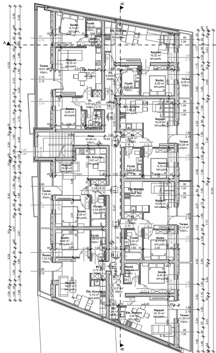
2. EMELETI ALAPRÁJZ 100 m
